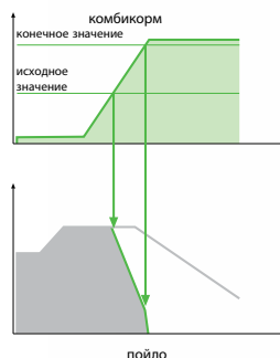
Схематическое изображение метода кормления в зависимости от комбикорма.
